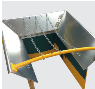
Ekstraleveä syöttölaite kottikärryille
